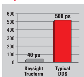
Jitter
